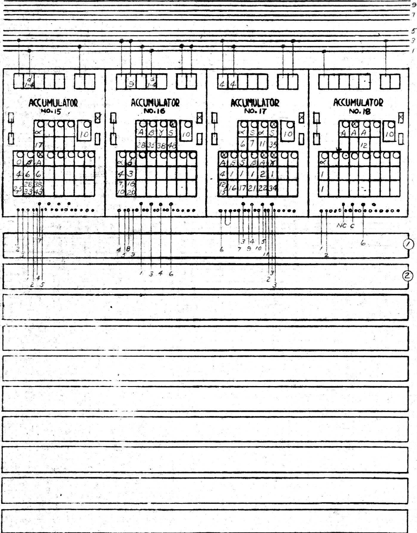
Fig. 7-3 (d) Quadratic Lagrangian Interpolation - Set-Up Diagram
